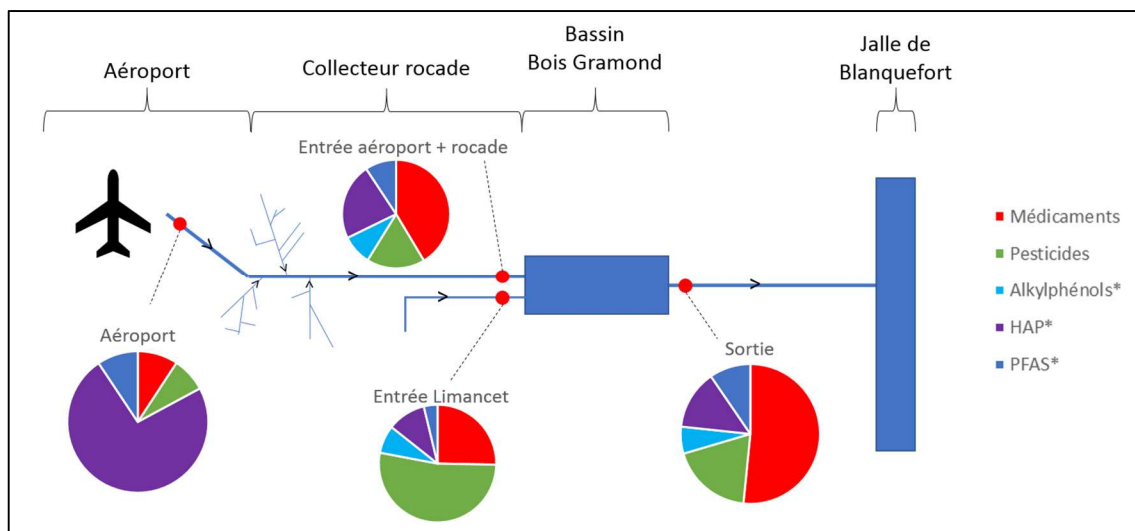
Figure 3. Représentation schématique du collecteur Rociade Nord et de l'empreinte en micropolluants des différents points de prélèvement.
