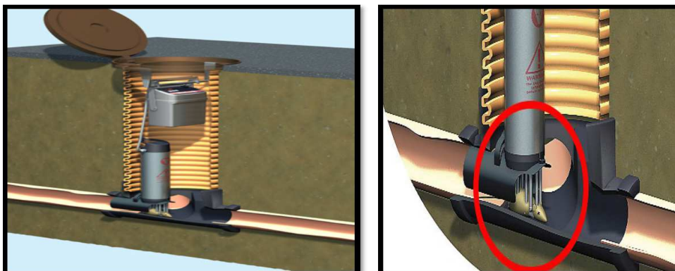
Figure 35 Exemple d'une technique mécanique(WiseCon®) permettant la dératisation des réseaux d'assainissement sans utilisation de produits chimiques.
