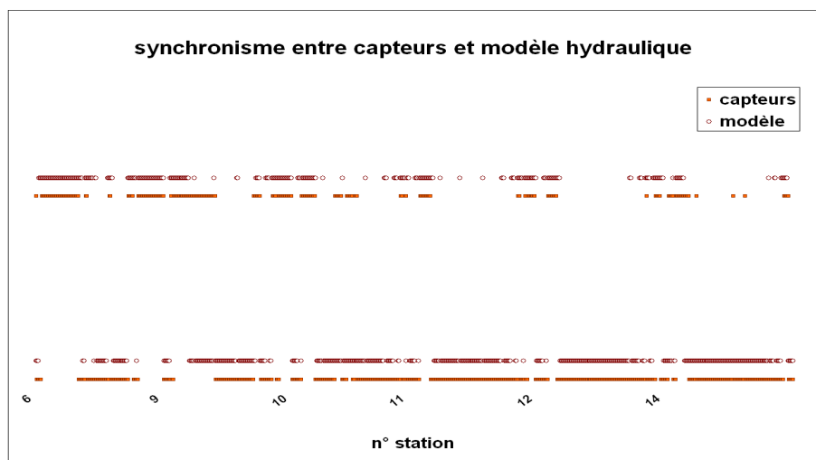
Figure 14 : Représentation du synchronisme entre périodes en eau (en haut) et en assec (en bas) des capteurs (lignes continues) et du modèle hydraulique (lignes à points)
