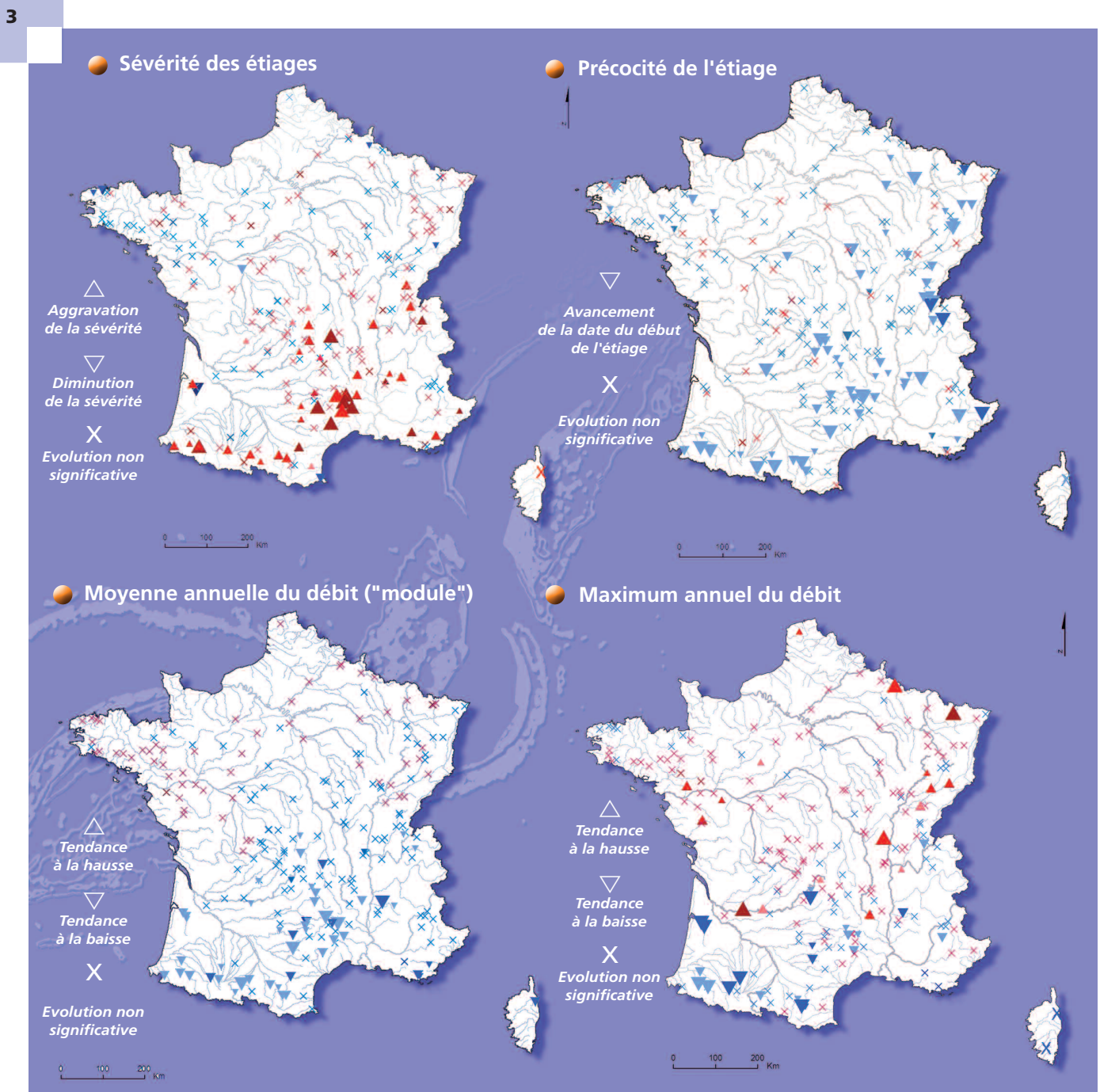
Figure 3. Tendances détectées de 4 indices : Sévérité des étiages - Précocité de l'étiage - Moyenne annuelle du débit - Maximum annuel du débit
