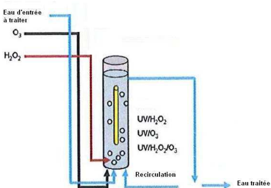
Figure 5 : Le réacteur photochimique du pilote POA
