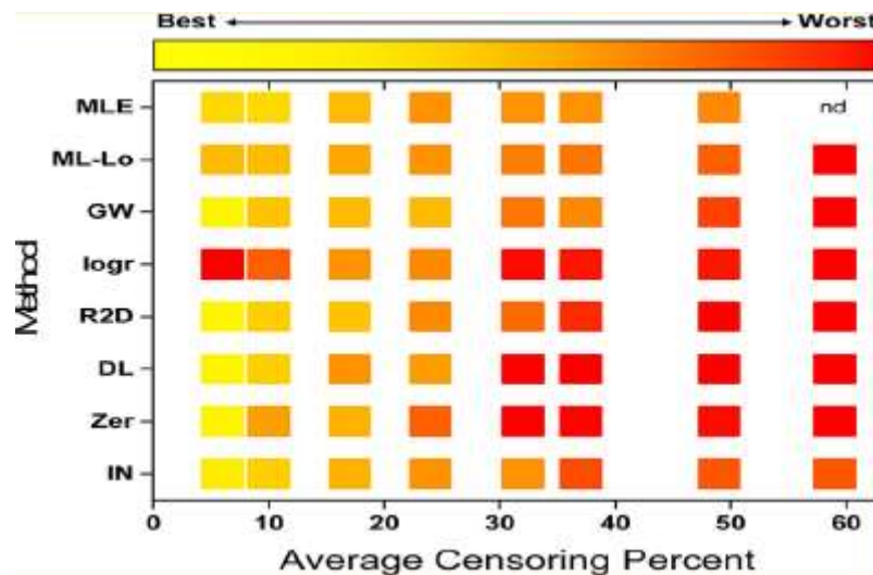
Figure 2 : Evaluation d'approche statistique pour traiter les données <LQ avec fiabilité (Antweiler, 2015)
