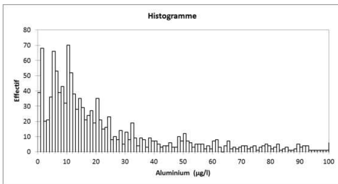
Figure 6 : Courbe de fréquence cumulée des médianes de concentrations en aluminium pour l'ensemble des qualimètres (axe coupé à 100 µg/L)- (LQ/2 max : 1,5 µg/L).
