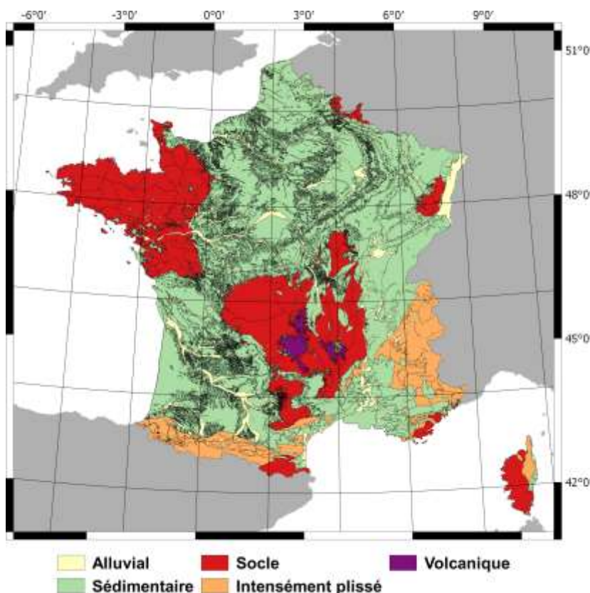
Figure 4 : Carte schématique de répartition des entités nationales de niveau 3 selon les types de formation géologique
