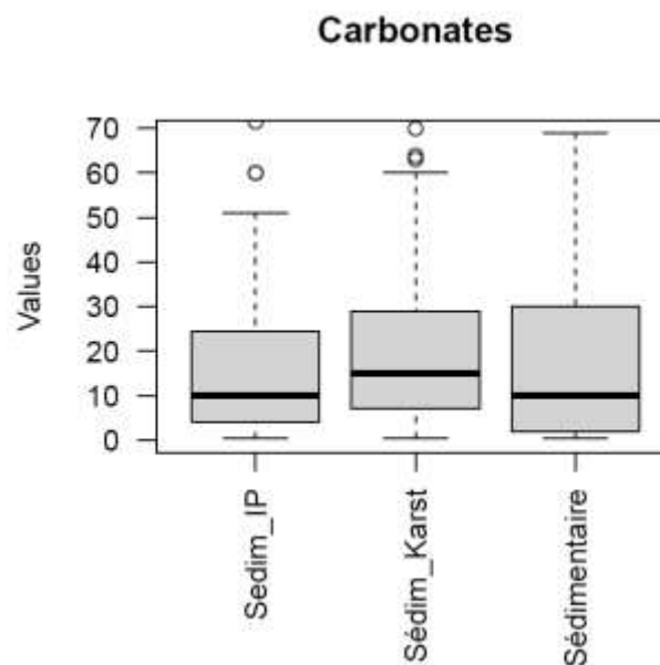
Figure 8 : Boîte à moustache pour les carbonates selon le domaine (IP :intensément plissé, karstique, bassin sédimentaire).
