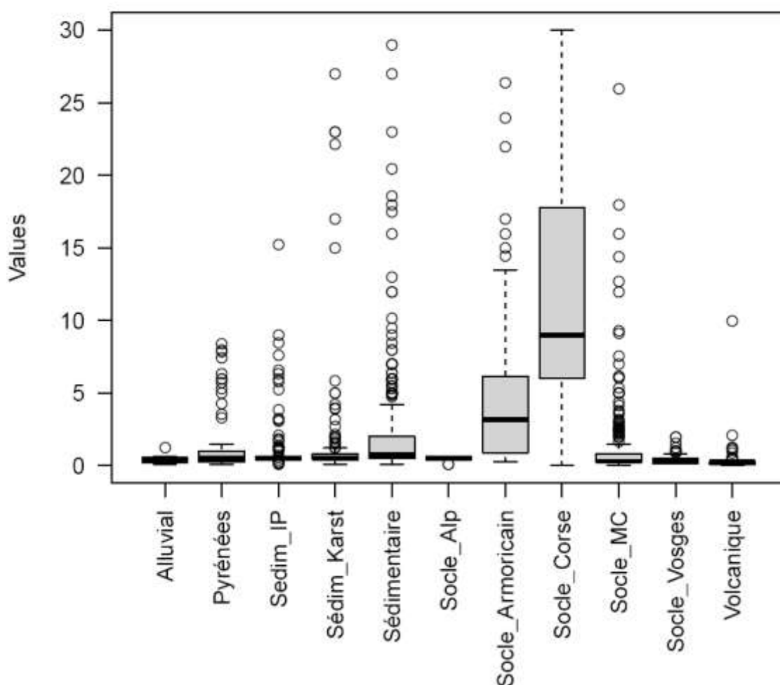
Figure 5 : Boîte à moustache des données utilisées pour l'étude statistique des concentrations en nickel selon les domaines investigués.
