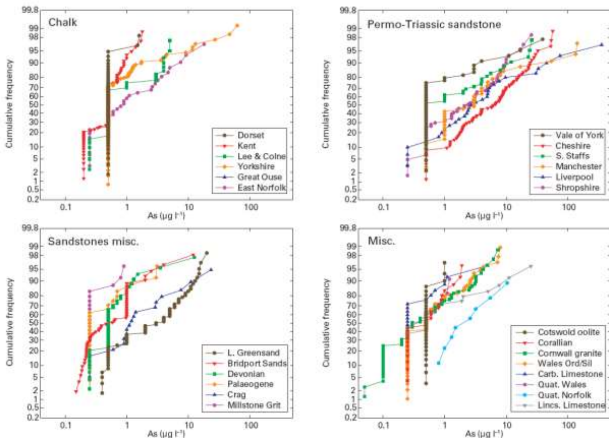
Figure 1 : Fréquence cumulée des concentrations en arsenic dans les eaux souterraines (Shand et al., 2007).
