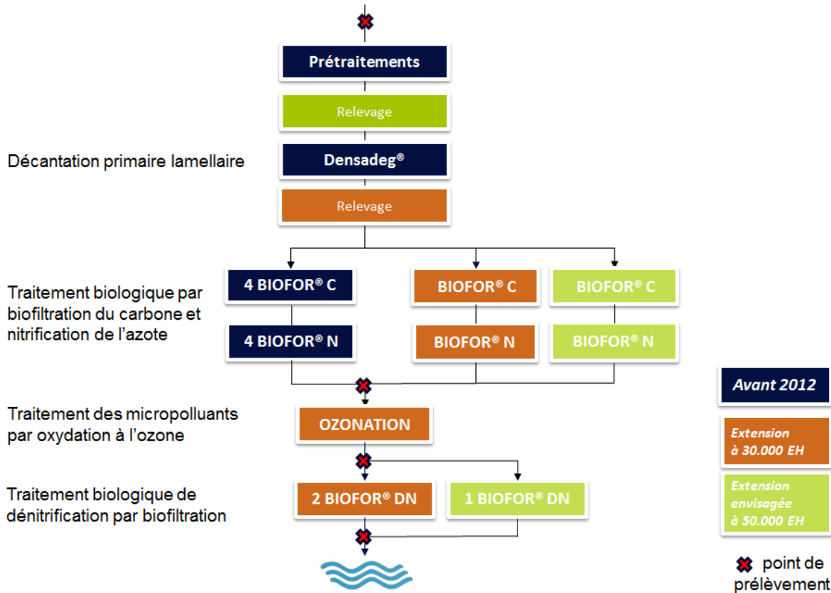
Figure 2. Représentation schématique de la filière de traitement des eaux de la station de Sophia Antipolis « Les Bouillides »
