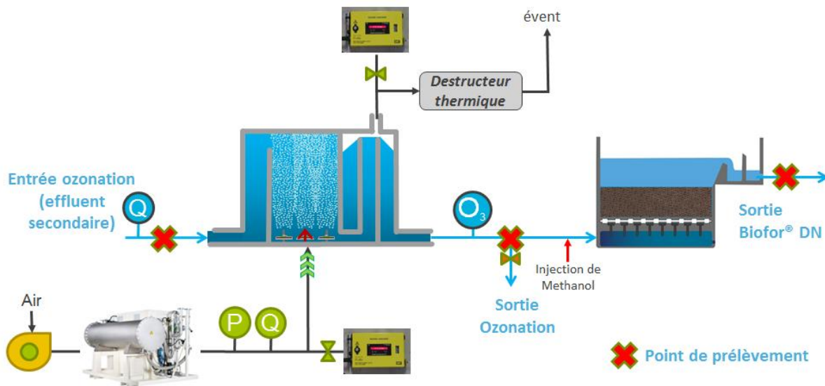
Figure 3: Représentation schématique du traitement complémentaire par ozonation de la STEU des Bouillides
