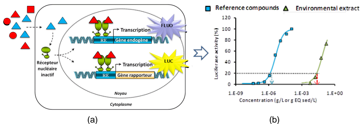
Figure 4. (a) Principe des bioessais in vitro utilisés pour la bio-détection des activités PE et HAP-like dans le projet MICROPOLIS et (b) exemple de courbes dose-réponses obtenues.
