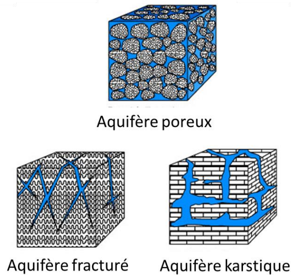
Figure 4. Trois différents types d'aquifères selon leur porosité/perméabilité (modifié d'après http://www.cima.ualg.pt/piloto/UVED_Geochemie/UVED/site/html/2/2-2/2-2-2/2-2-2-2.html )
