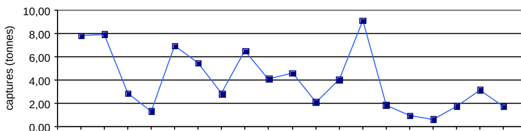
Évolution de captures de civelle par les marins pêcheurs dans l'estuaire de l'Adour (dans la partie salée et en eau douce) [source Cereca – Institution Adour, 2007]
