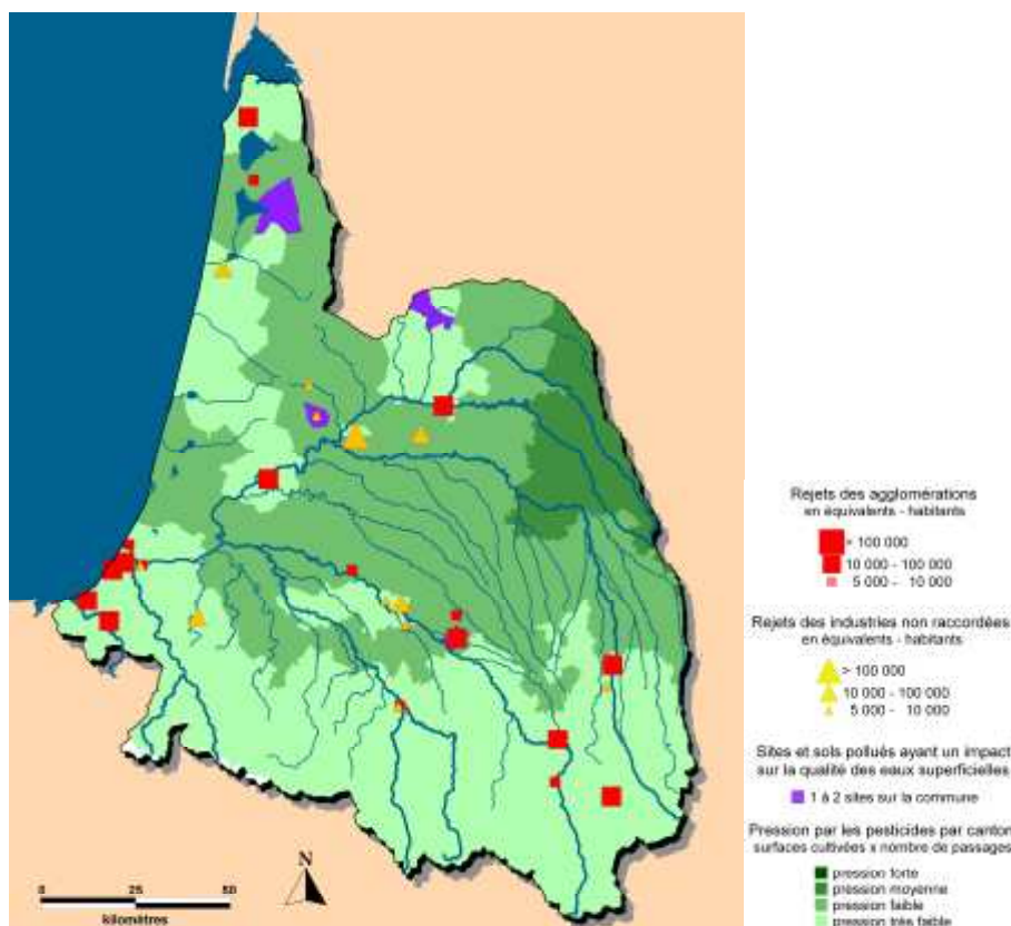
Principales sources de pollution potentielles urbaines industrielles et agricoles sur le bassin Adour et cours d'eau côtiers (source état des lieux du SDAGE Adour Garonne)
