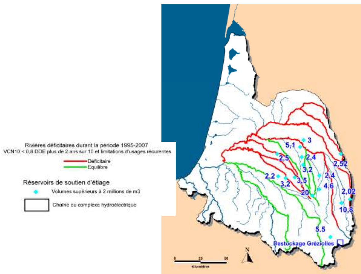
Rivières déficitaires et réserves de soutien d'étiage sur le bassin Adour et cours d'eau côtiers (source état des lieux du SDAGE Adour Garonne)
